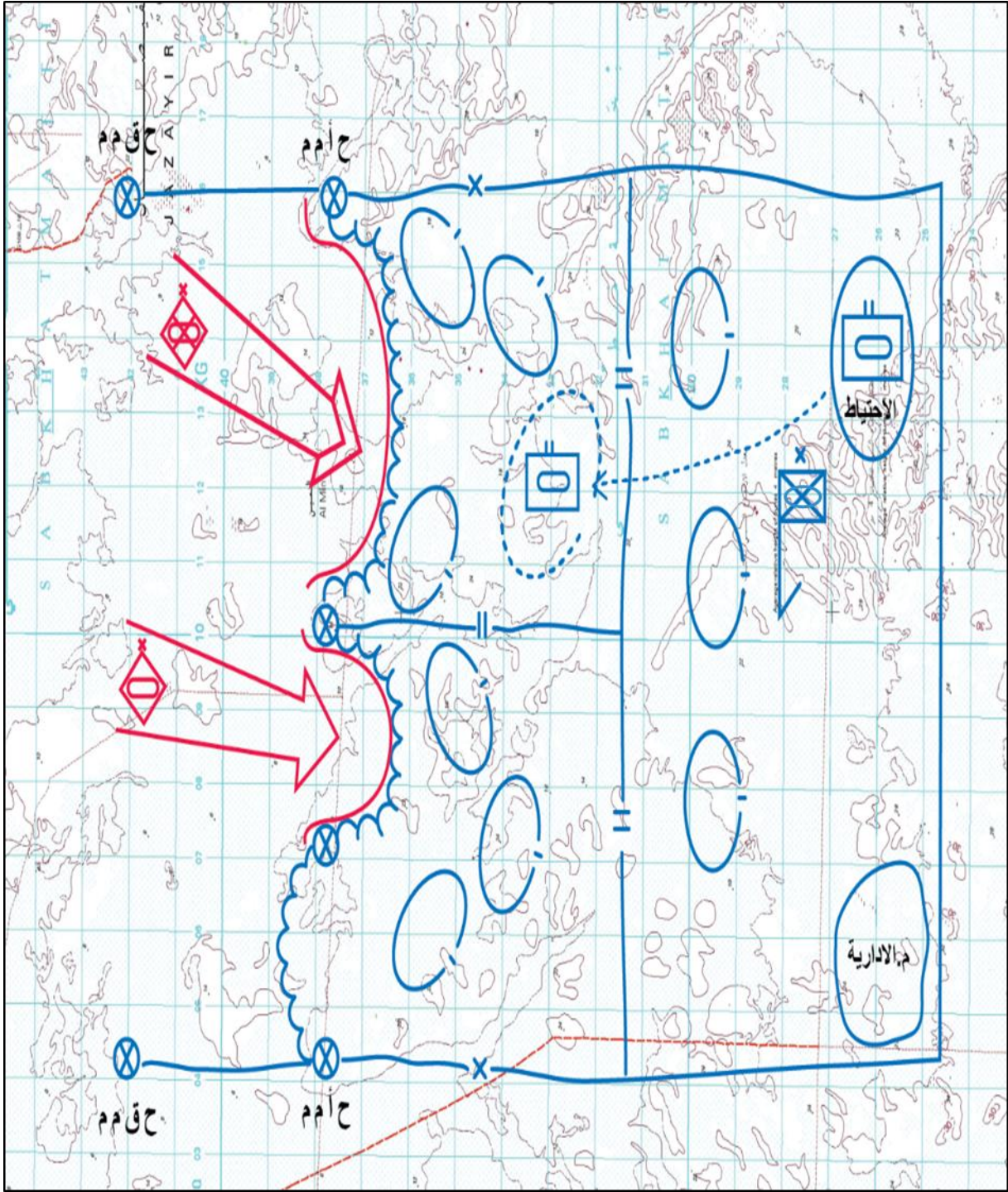
الشكل رقم (8) مجموعة اللواء تعزز بالاحتياط موقع الإختراق الأكثر خطورة
