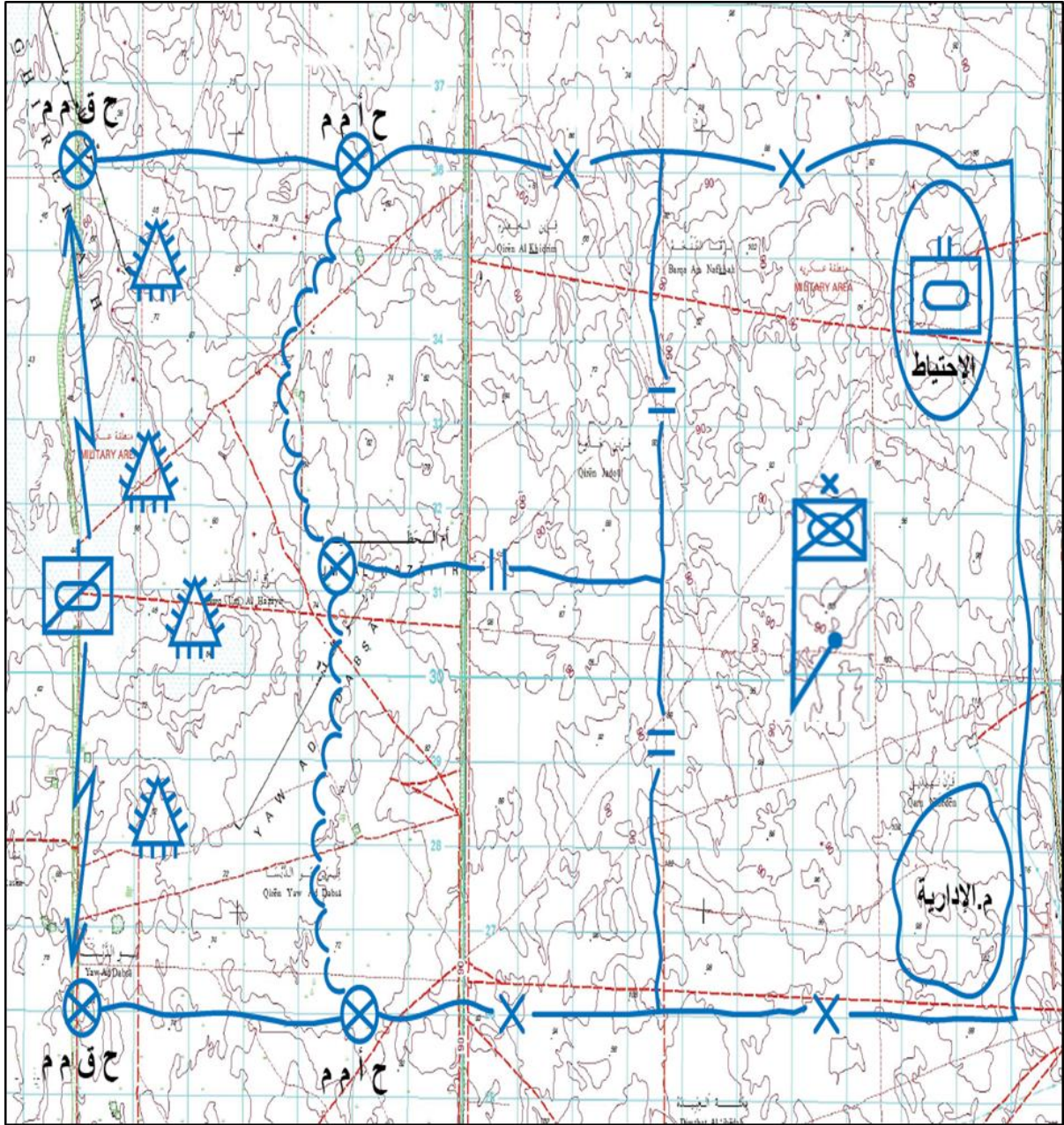
الشكل رقم (4) فصائل تعمل كنقاط قتال خارجية لمجاميع القتال/ الكتائب الأمامية
