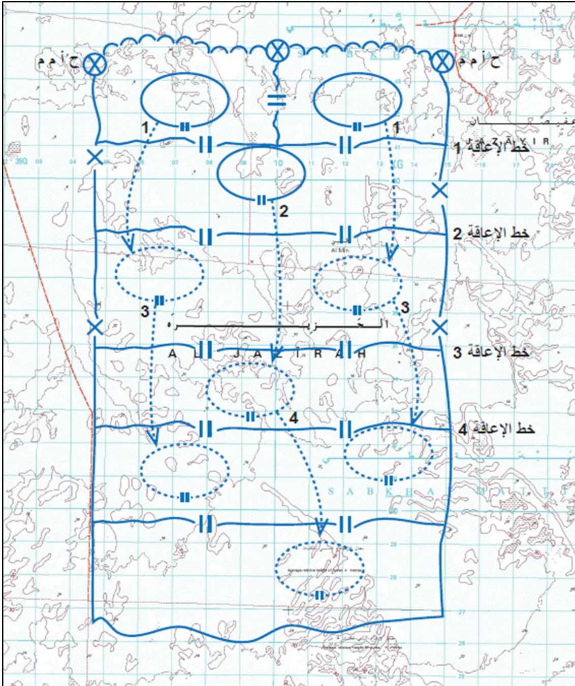
الشكل رقم (12) أسلوب الإعاقة التبادلية
